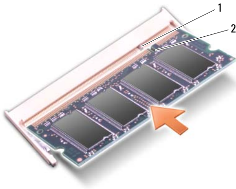
1 卡舌 2 槽口
